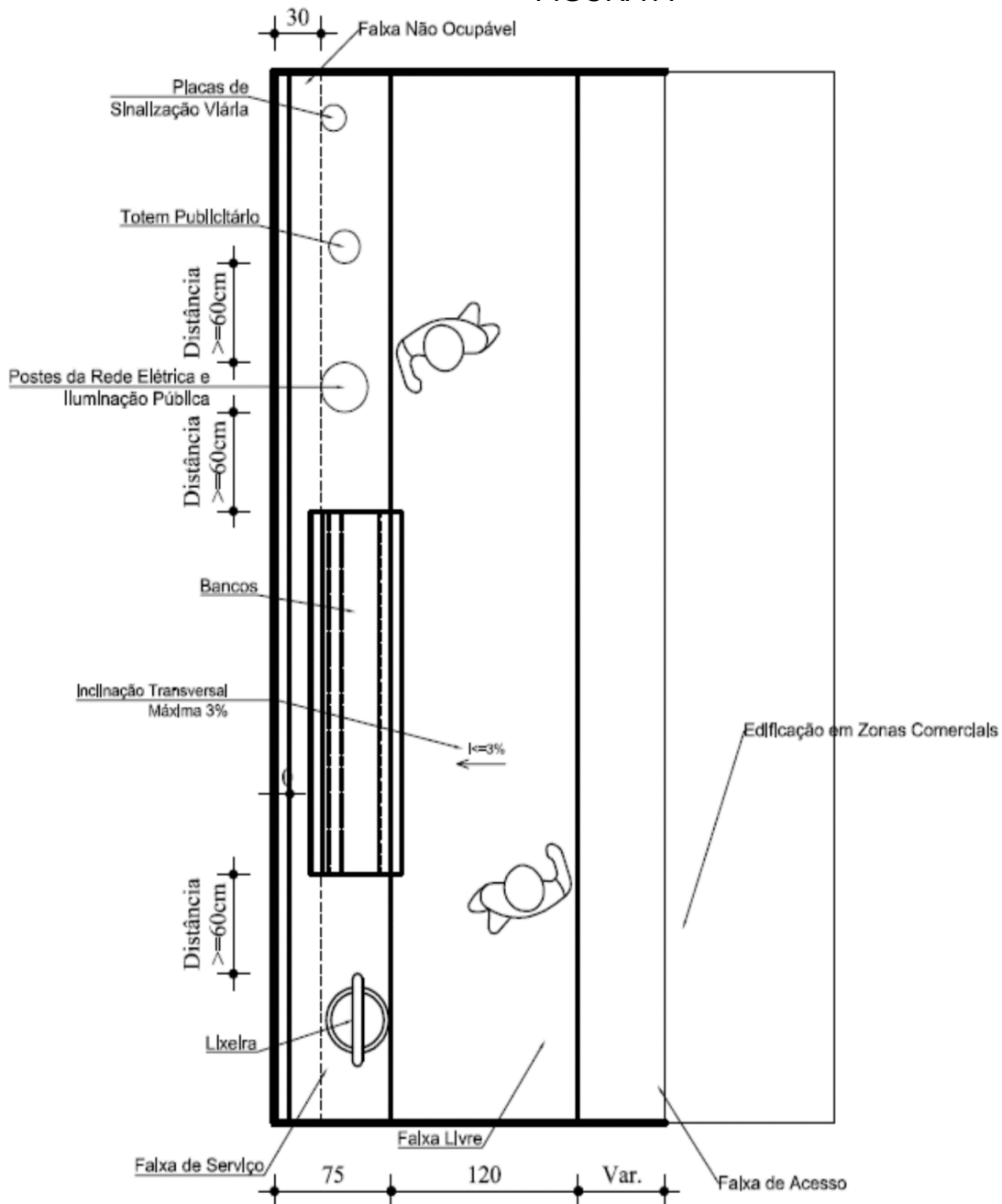
Planta Baixa
